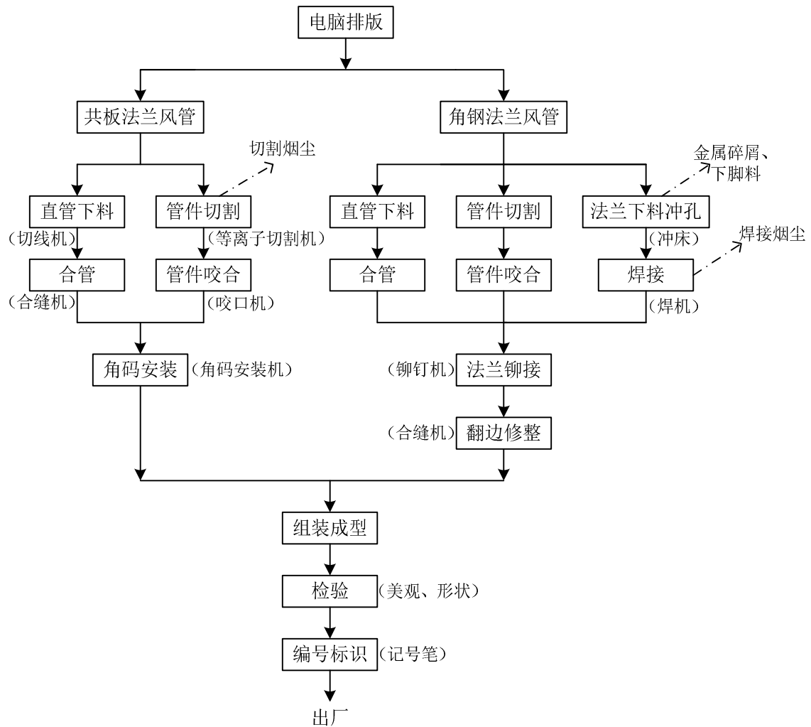
图 5-2 风管生产工艺流程及产污图
