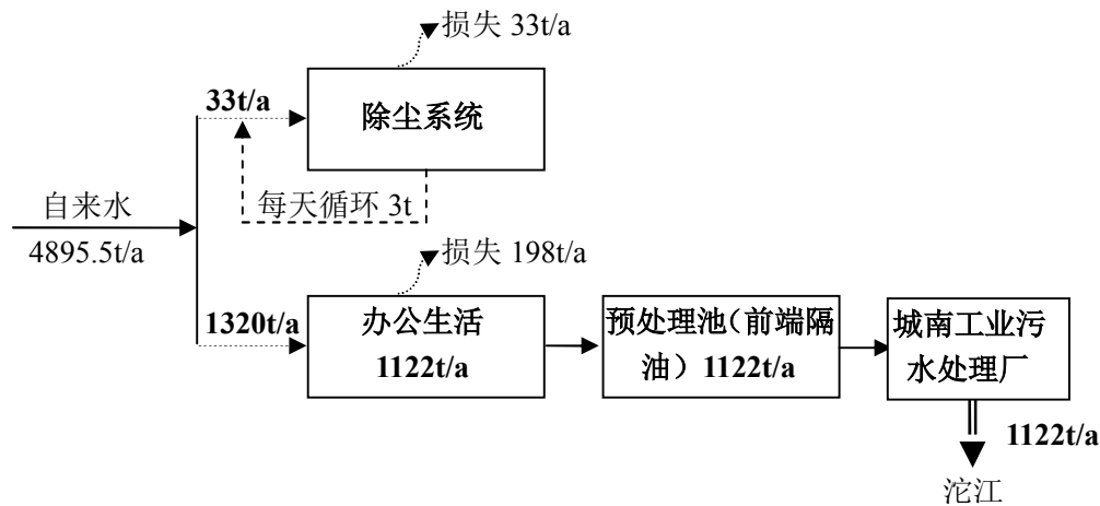
图 5-4 项目水平衡图(t/a)
